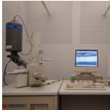
Microscopio electrónico de barrido del IAPH / EUGENIO FERNÁNDEZ RUIZ, IAPH
