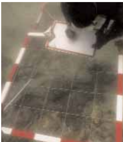
➤ Registro gráfico de estructura naval de un navío de línea (Cádiz) / J.M. HIGUERAS
