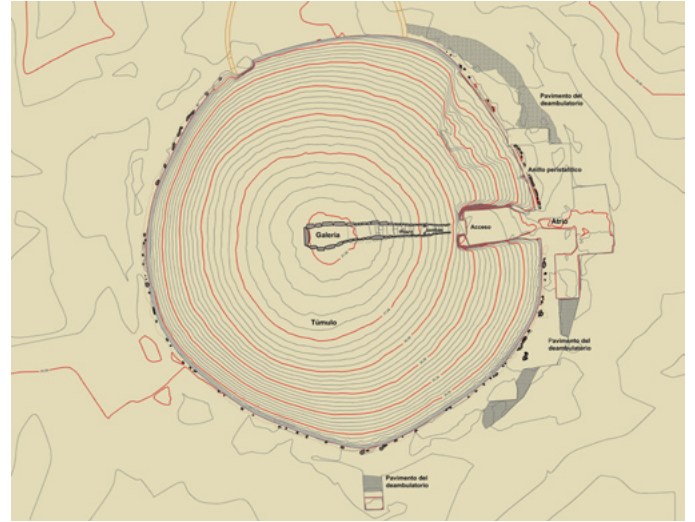
5. Planta de los elementos arquitectónicos que conforman el dolmen
