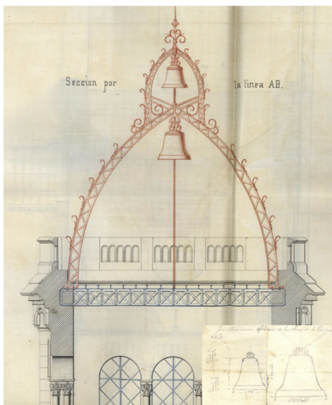
Elias Rogent. Sección de la Torre de Letras con la modificación para la espadaña y las dos campanas (1877) | fuente Archivo Histórico de la Universidad de Barcelona
